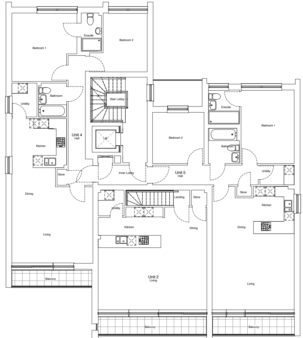
Grd Floor GA 1 : 50
